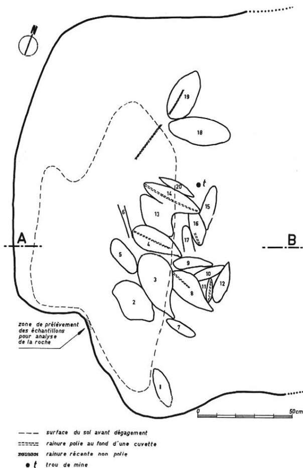
Fig. 7 : Palluau-sur-Indre (n° 55). La zone fonctionnelle (Relevé J.-L. Girault, mise au net P. Trotignon).
